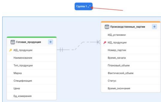
Рисунок 30 - Работа с группами в логической модели
