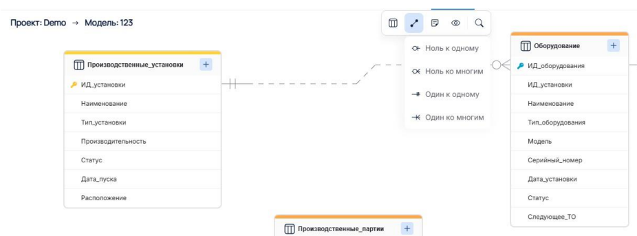
Рисунок 27 - Создание связи
