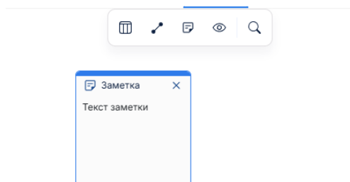
Рисунок 29 - Добавление заметок
