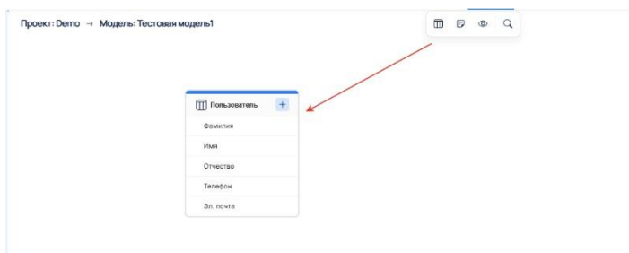
Рисунок 25 - Создание таблицы
