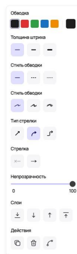
Рисунок 13 - Настройка связей
